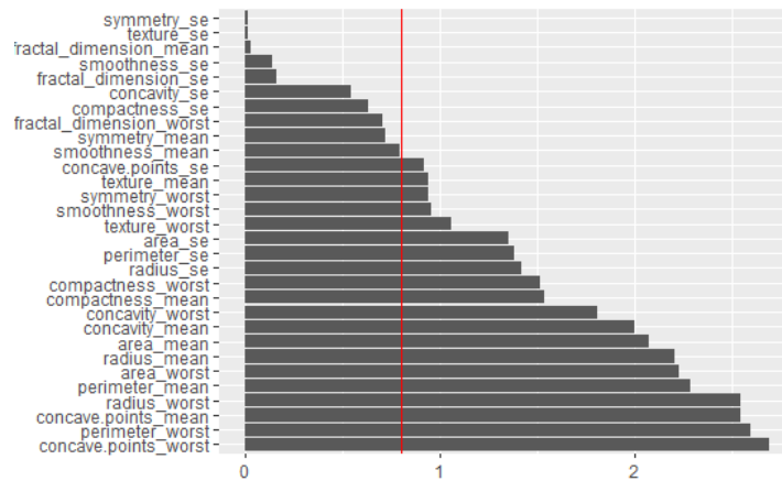
(a) Pesos de cada característica d de Cohen. La línea roja corresponde a un valor d = 0,8
