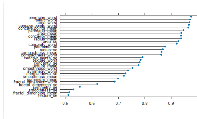
(b) Pesos de cada característica LVQ
