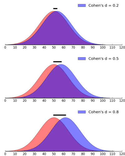
Figura 3: Tamaño del efecto para diferentes d de Cohen para dos clases. Observe que a mayor valor d , mayor es la diferenciación entre las clases.
