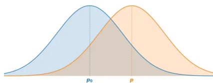
Figura 1: Comportamiento de una variable para dos grupos o clases distintas, color azul para la clase benigna y color amarillo para la clase maligna. Observe como las medias p_0 y p , se pueden diferenciar claramente entre sí.
