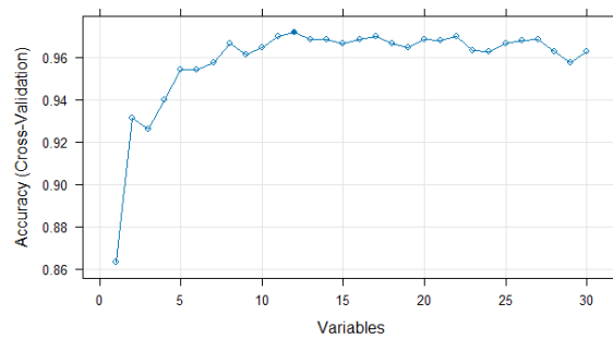
Figura 8: Subconjunto de las 12 características óptimas usando RFE.
