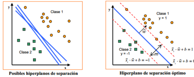
Figura 5: Hiperplano de separación en un espacio bidimensional
