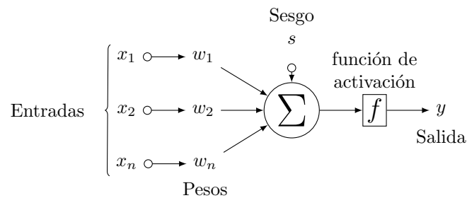
Figura 4: Diagrama de la arquitectura LVQ. Las entradas x corresponden a las características, el sesgo desplaza el resultado obtenido a través de la función de activación, la cual es lineal para LVQ, la salida y puede ser y = 1 para la clase M o y = 0 para la clase B
