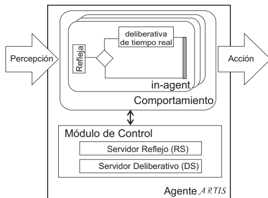
Figura 3.1. Arquitectura de Agente ARTIS: Modelo de Usuario
