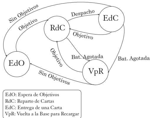
Figura 5. Autómata Finito No Determinista de Comportamientos
